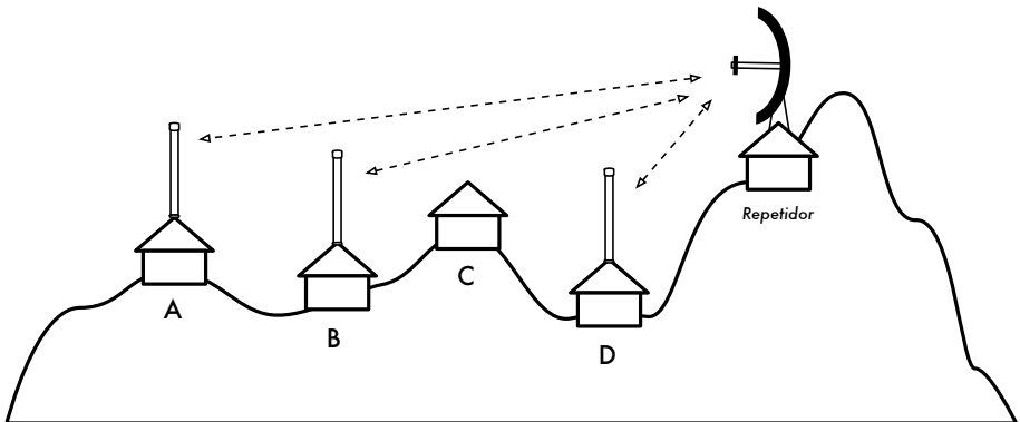
Figura 3.13: El lugar D no puede ver al lugar A o al B, porque el lugar C está en el camino y no está interesado en tener un nodo. Al instalar un repetidor en un lugar alto los nodos A, B, y D se pueden comunicar. El tráfico desde el nodo D en realidad viaja más lejos que el del resto de la red antes de que el repetidor reenvíe esos datos.
