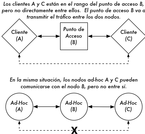
Figura 3.7: El punto de acceso B va a transmitir el tráfico entre los clientes A y C. En el modo ad hoc , el nodo B no va a transmitir el tráfico entre A y C por omisión.
